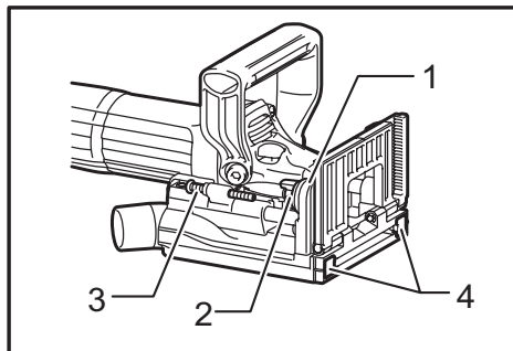
► 1. Index 2. Butoir 3. Vis de réglage 4. Crampon en caoutchouc
