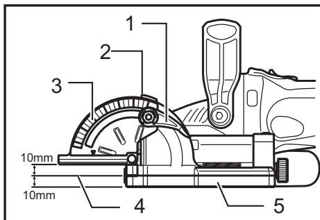
► 1. Levier de verrouillage 2. Index 3. Secteur angulaire 4. Plan médian de l'épaisseur de la lame 5. Couverture de lame
