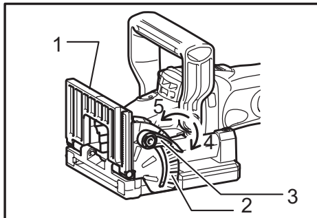
► 1. Plaque frontale 2. Secteur angulaire 3. Levier de verrouillage 4. Serrer 5. Desserrer
