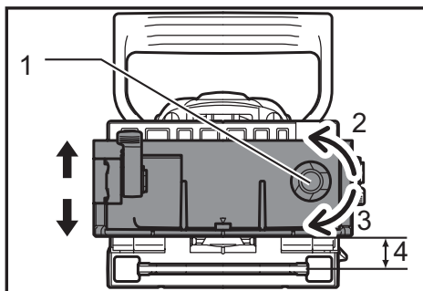
► 1. Bouton 2. Pour descendre 3. Pour monter 4. Plan médian de l'épaisseur de la lame
