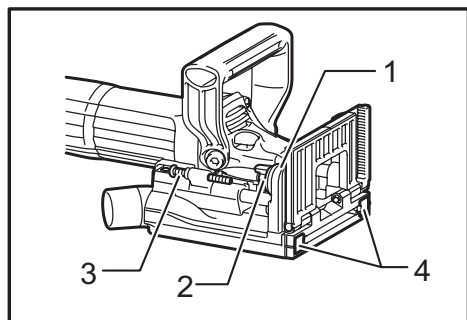
► 1. Puntero 2. Tapón 3. Tornillo de ajuste 4. Punta de hule
