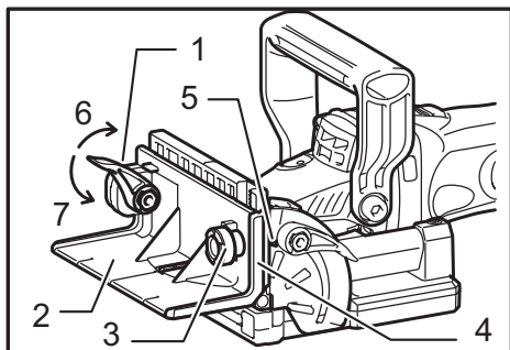
► 1. Levier de verrouillage 2. Guidage d'angle 3. Bouton 4. Échelle 5. Index 6. Serrer 7. Desserrer
