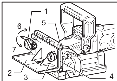
► 1. Palanca de bloqueo 2. Guía de ángulo 3. Perilla 4. Escala 5. Puntero 6. Apretar 7. Aflojar
